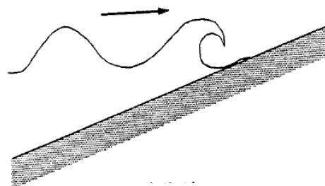
図2 巻き波
